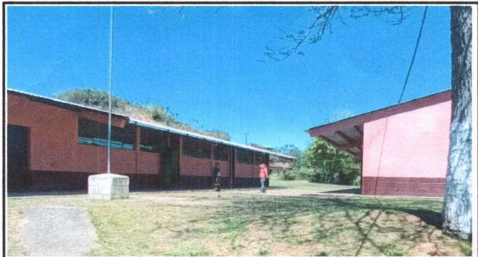
Foto 4. MODULO 2: Mejoramiento de entechado de pasillo entre aulas de dicho módulo.
