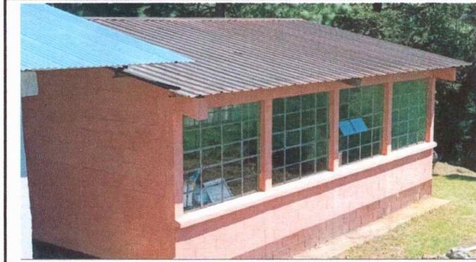
Foto 1. MODULO 1: Cambio de entechado, instalación de canales e instalación de balcones.
