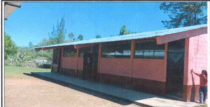
Foto 6. MODULO 2: Reparación y ampliación de techo y piso de pasillo.
