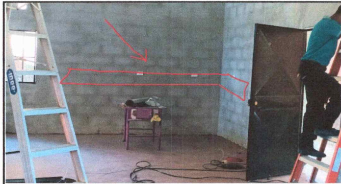
Foto 3. MODULO 1: Instalación de desayunador dentro de cocina e instalación de balcones.
